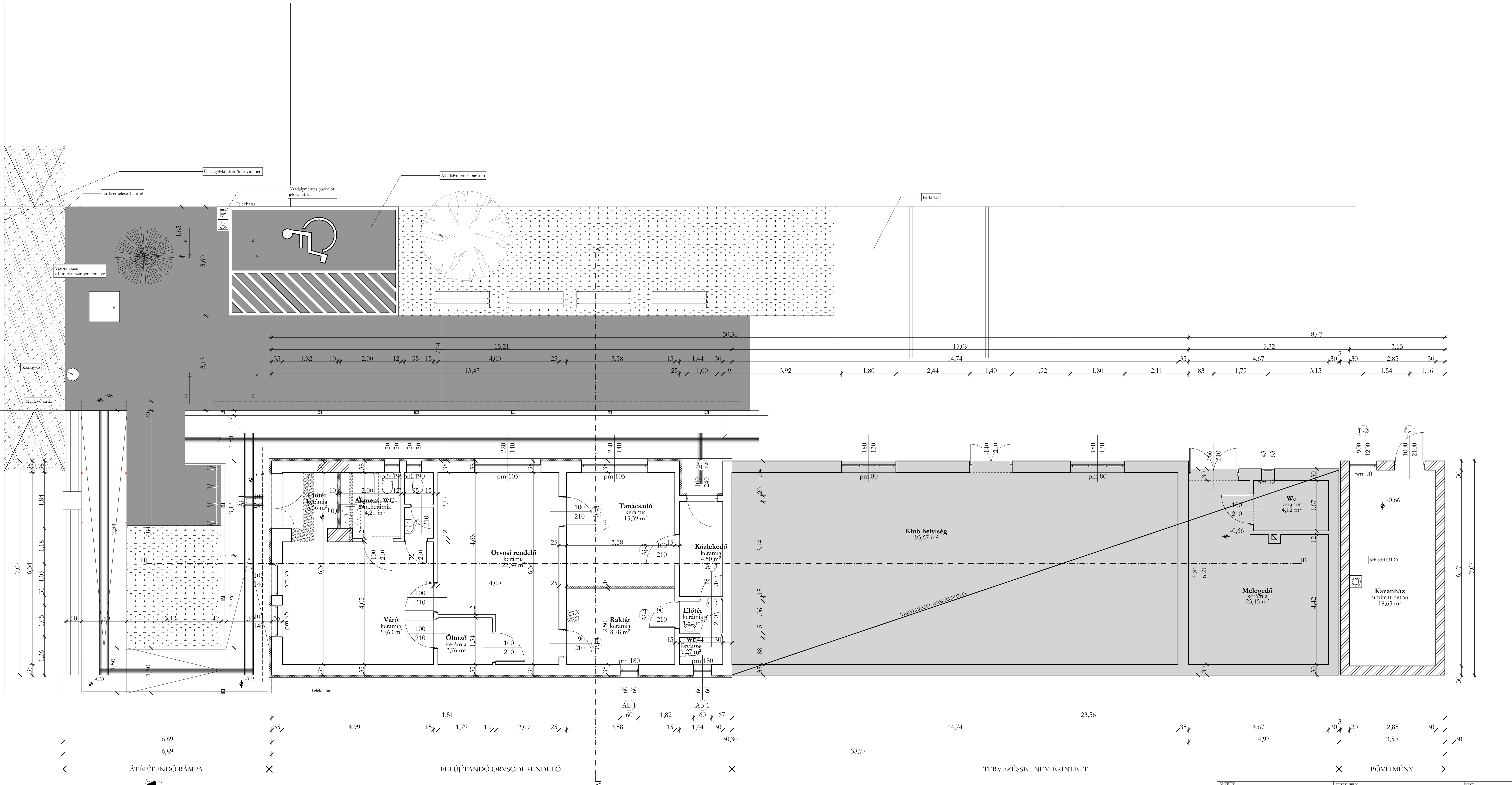
ALAPRAJZ M=1:50
