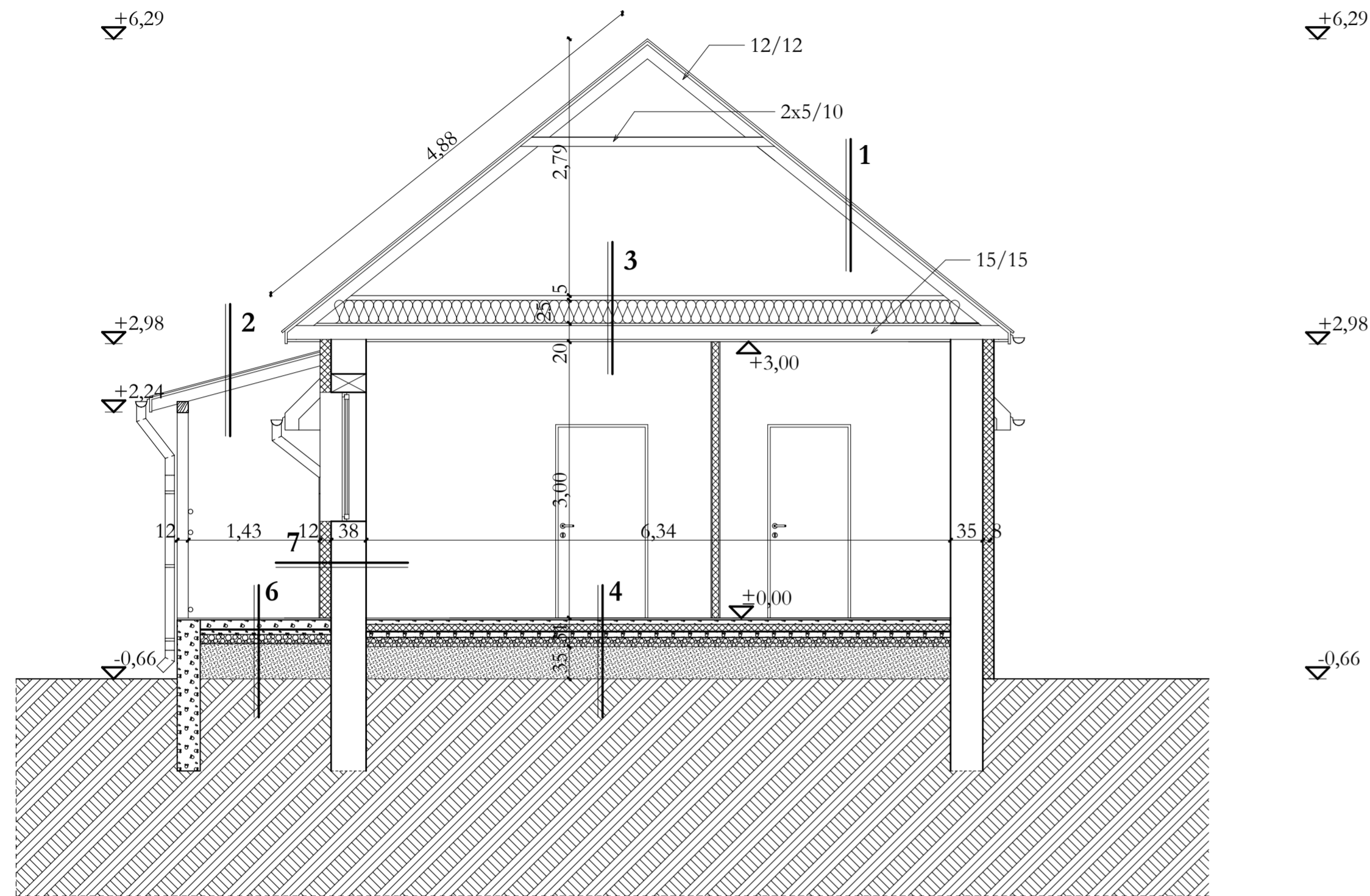
A-A METSZET M=1:50
